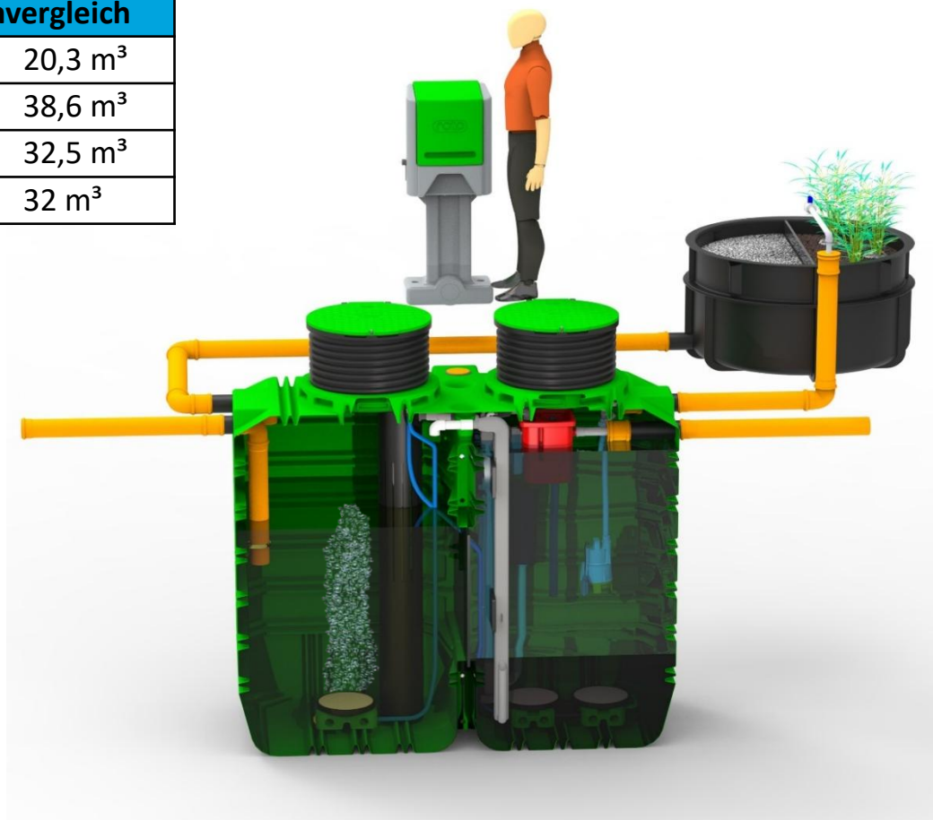
Beispielbild: BioTopp Kleinkläranlage für 14 Personen in einem 6 m 3 Kunststoffank
