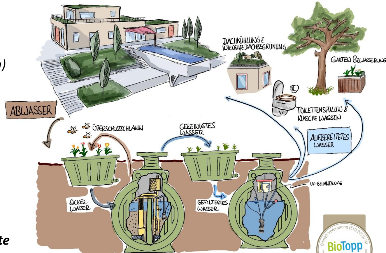
Schematische Darstellung BioTopp Wasserwiederverwendungssystem
