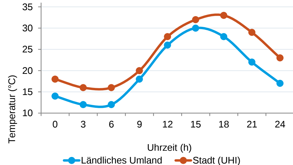
Tagesgang: Stadt bleibt nachts warm (schematisch)
